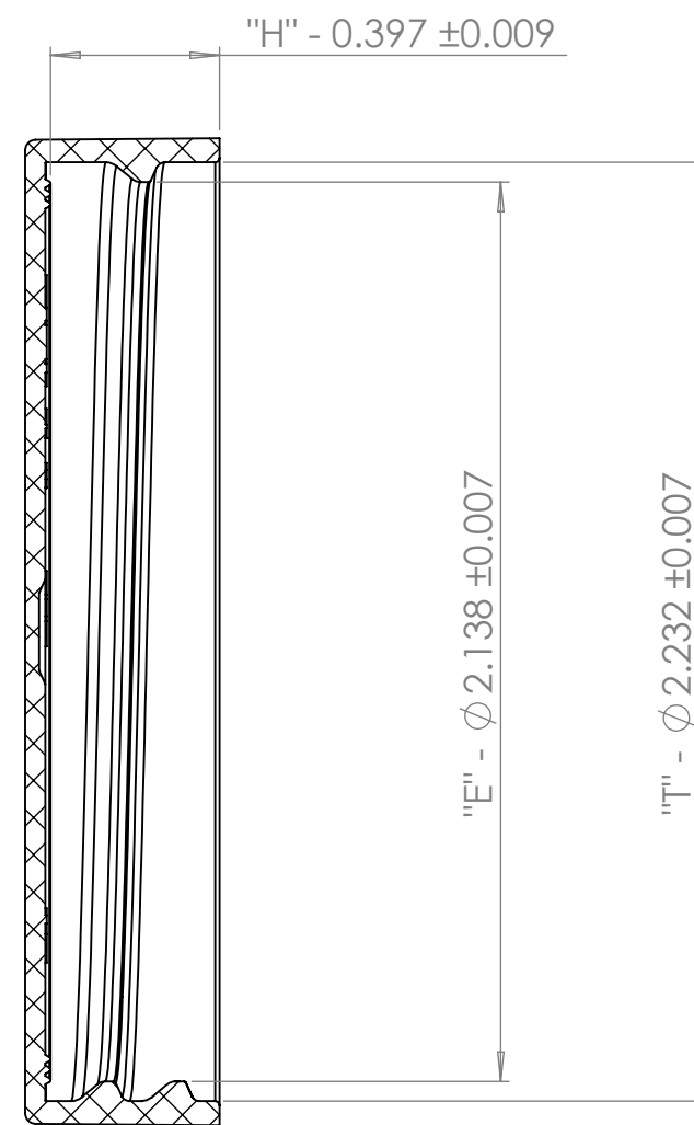
SECTION A-A
